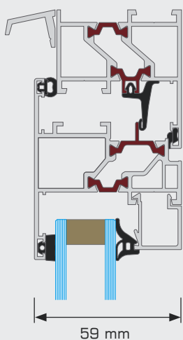
przekrój pionowy okna
