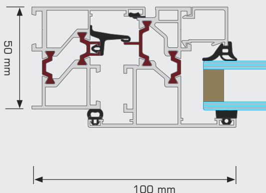
przekrój poziomy okna
