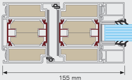
przekrój drzwi EI 45, EI 60
