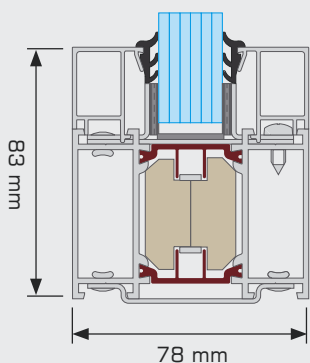
przekrój przez ściankę stałą EI 15, EI 30
